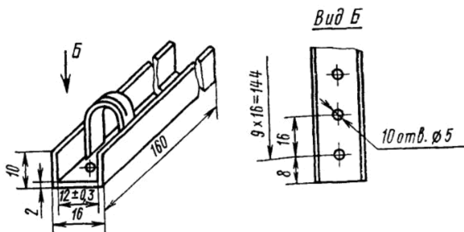
Держатель для образцов
