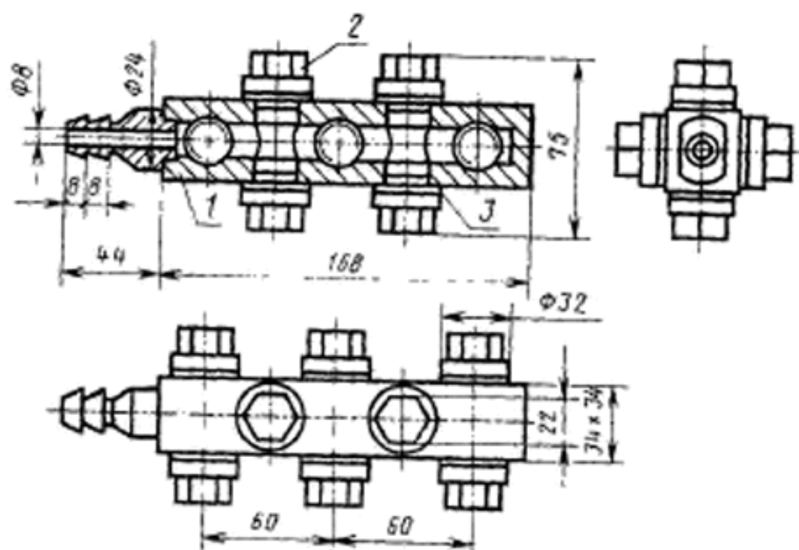
1—корпус; 2—заглушка; 3—фибровое уплотнительное кольцо
