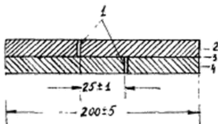
1—прорезы; 2, 4—слой фибры; 3—клеевой шов
