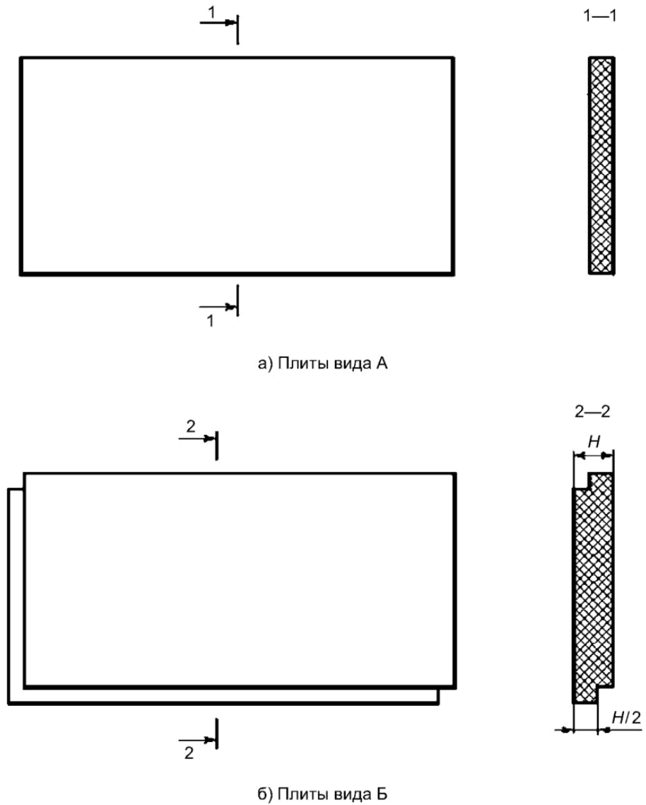
Рисунок Б.1 — Виды пенополистирольных плит
