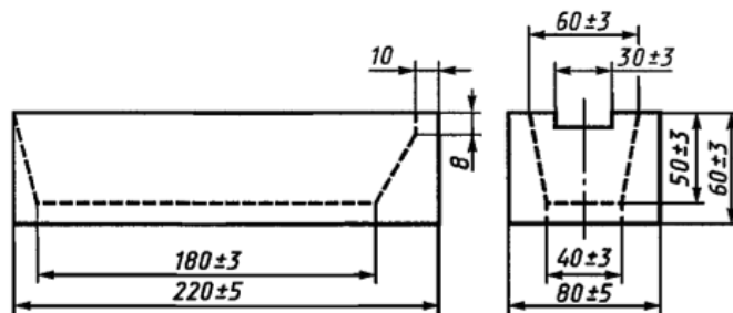
Рисунок 1 — Изложница
