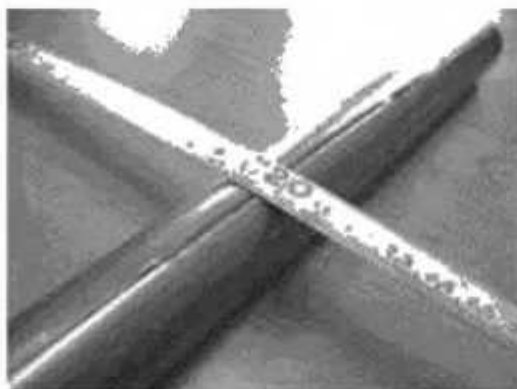
Трещина продольная на полуфабрикате
