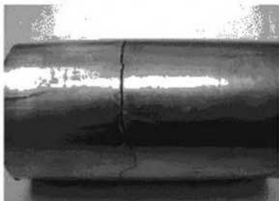
Трещина поперечная на полуфабрикате
