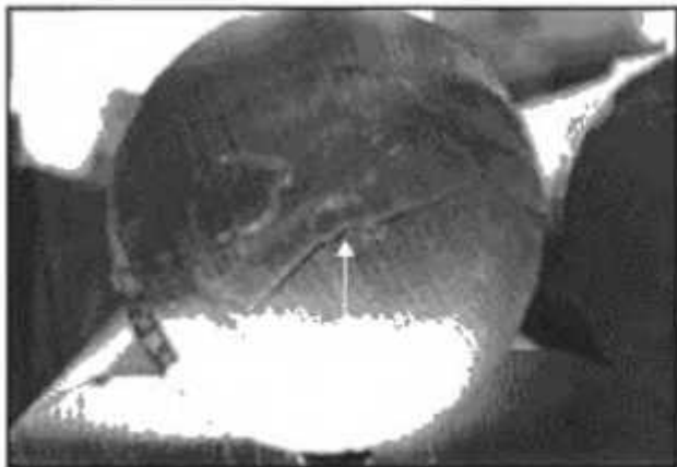
Трещина центровая на слитке
