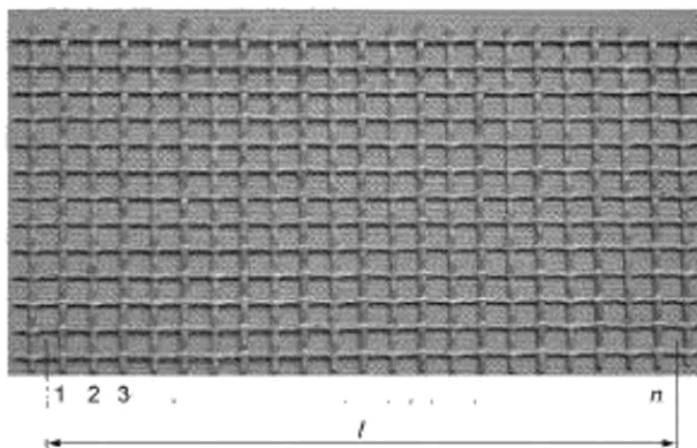
Рисунок 1 — Определение числа нитей
