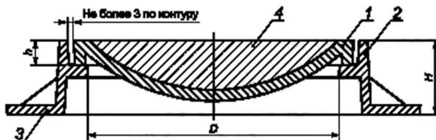
1 — крышка; 2 — корпус; 3 — опорная поверхность корпуса; 4 — бетон
