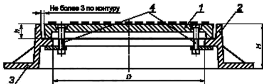
1 — крышка; 2 — корпус; 3 — опорная поверхность корпуса; 4 — замковое устройство
