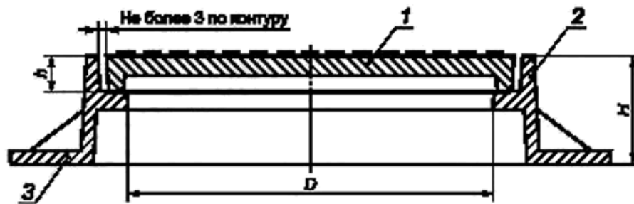
1 — крышка; 2 — корпус; 3 — опорная поверхность корпуса
