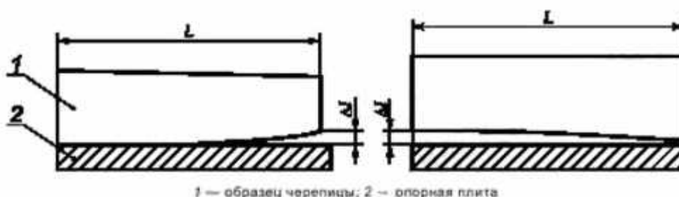
Рисунок 2 — Пример определения прямолинейности ребер черепицы
