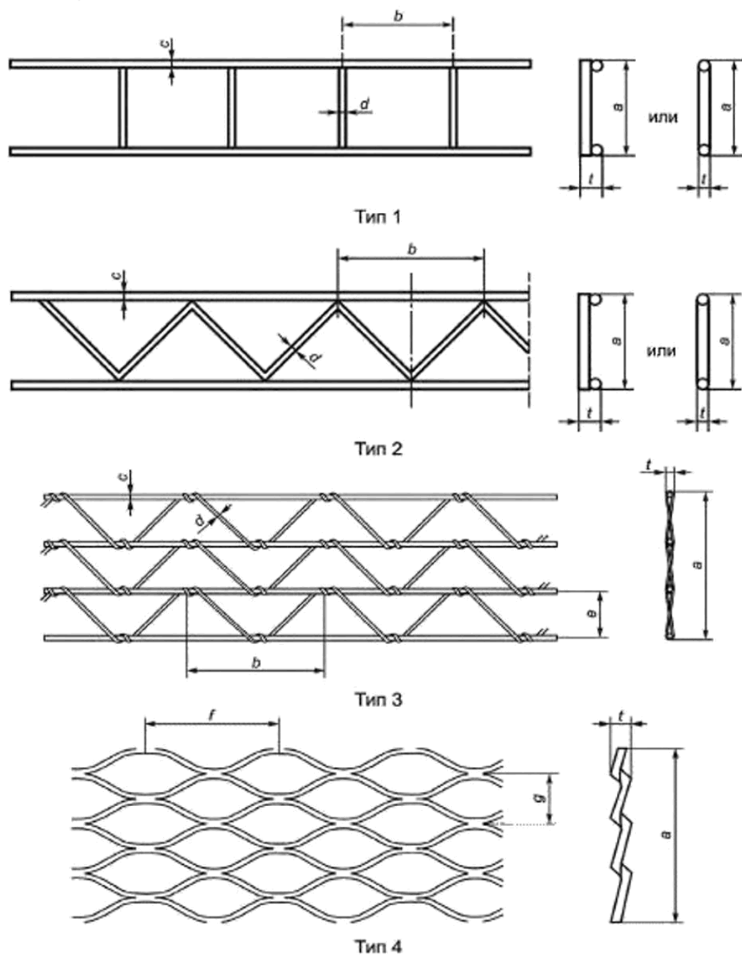
Рисунок 1 — Типы сеток
