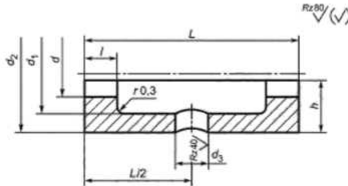
Рисунок Б.19 — Полушфита Пм для звеньев Ров грузоподъемностью свыше 2,00 тс
