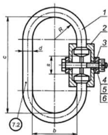
1 — скоба; 2 — полумуфта (2 шт.); 3 — кольца; 4 — Болт по ГОСТ 7798; 5 — гайка по ГОСТ 5919; 6 — шплинт по ГОСТ 397
