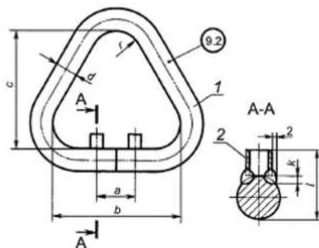
1 — скоба, 2 — упор (2 шт.)
