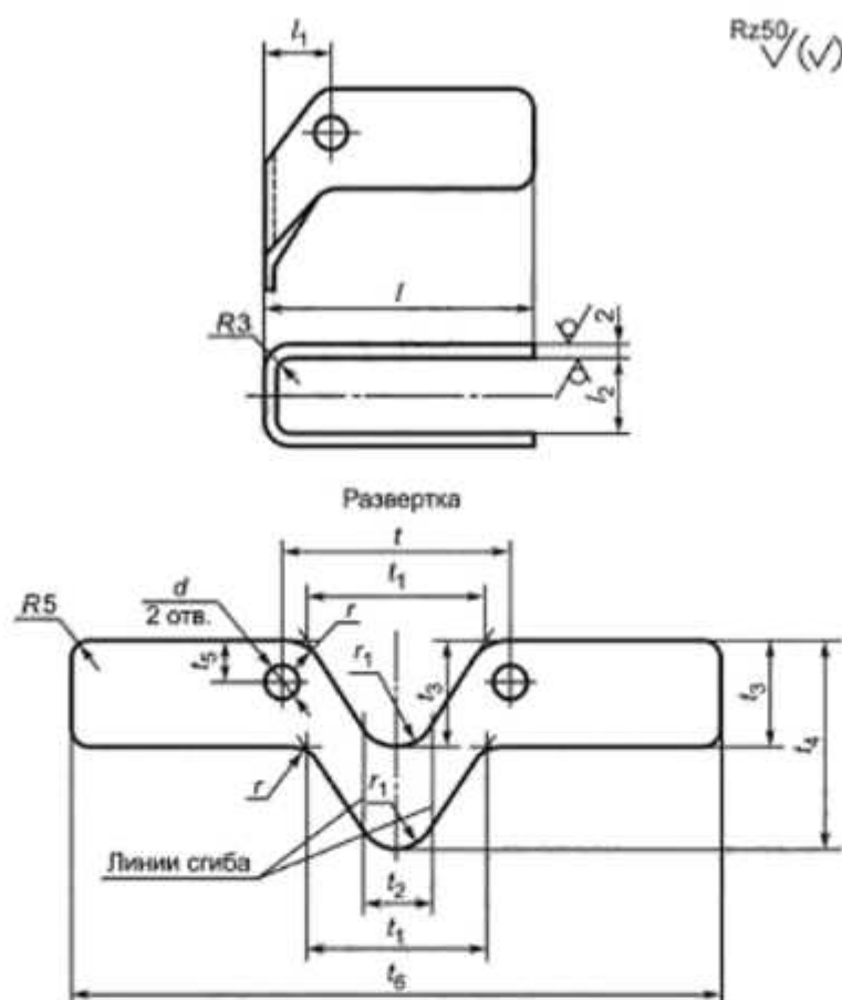
Рисунок Б.33 — Замок 31 для захвата К1
