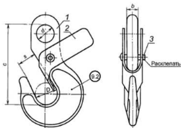
1 — крюк чалочный; 2 — замок; 3 — заклепка
