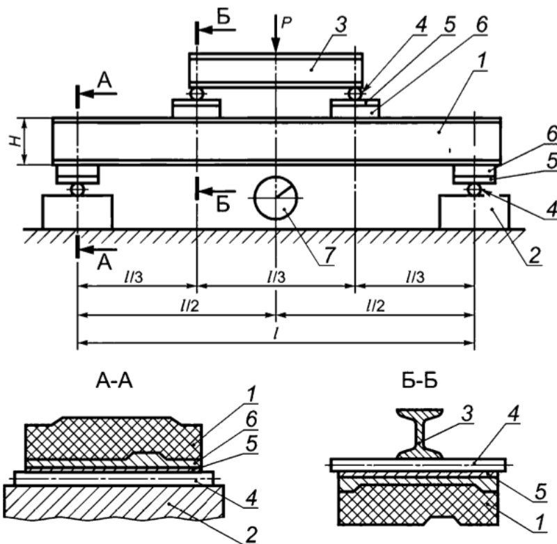
1 — образец; 2 — база; 3 — траверса; 4 — стальные цилиндрические опоры; 5 — стальные пластины; 6 — прокладки; 7 — прибор для измерения деформаций
