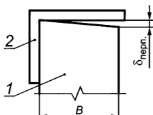
1 — панель; 2 — поверочный угольник 90^\circ ; B — ширина панели
