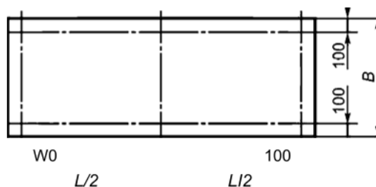
Рисунок 7 — Расположение мест проверки неплоскостности панели
