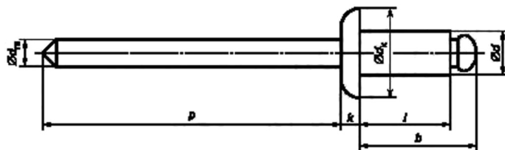
Рисунок 1 — Размеры заклепок
