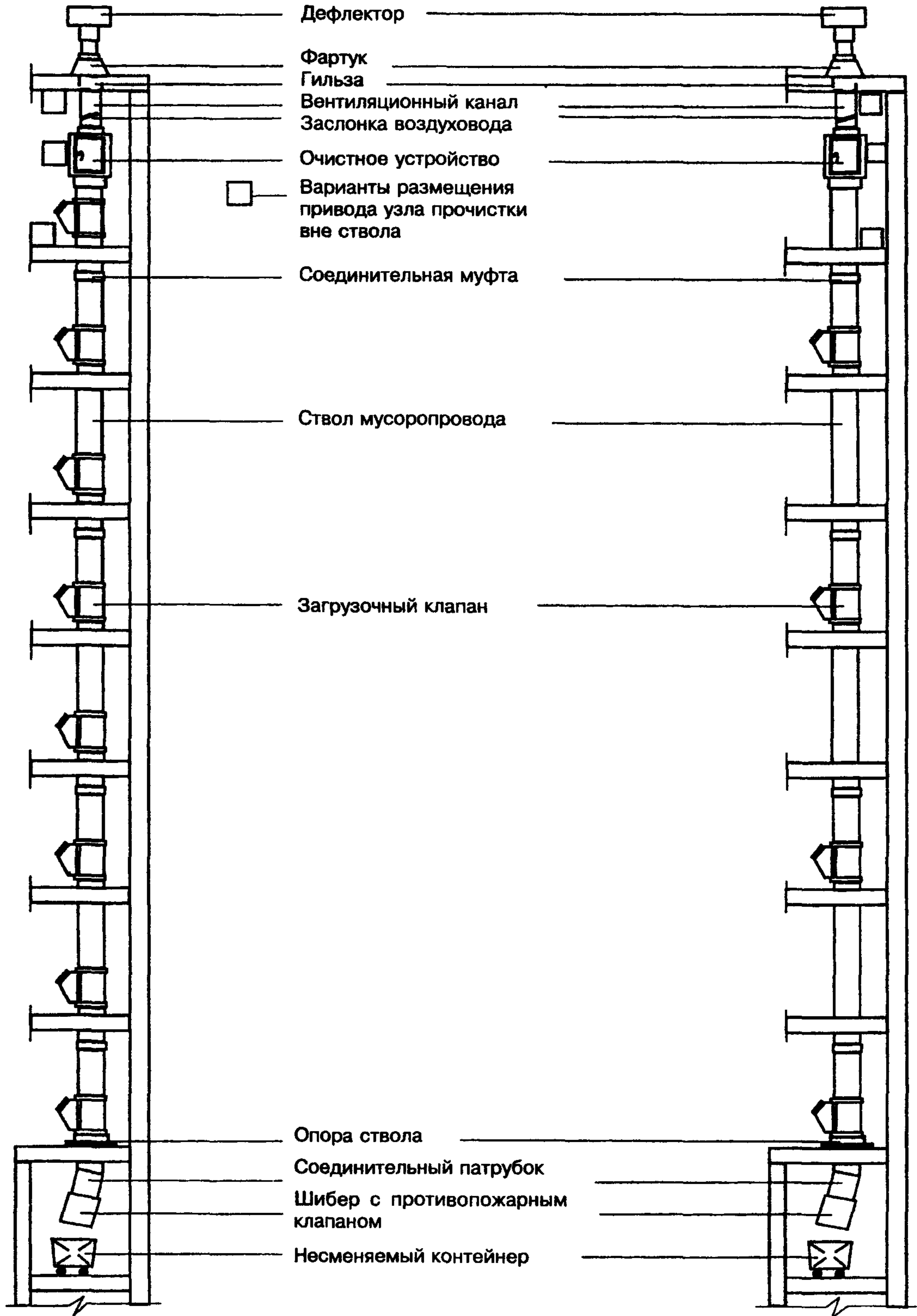
Вариант размещения загрузочных клапанов на поэтажных лестничных площадках
